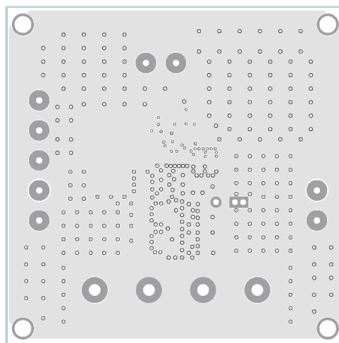
Inner1 Layer
