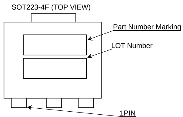
SOT223-4F
