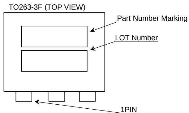
TO263-3F
