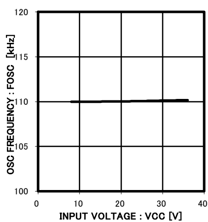
Fig.17 fosc-INPUT VOLTAGE
