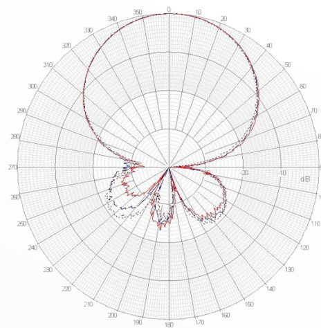
R2T9-12 E-Plane
