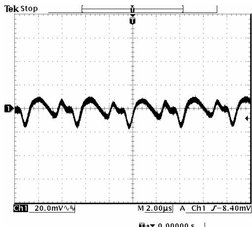
Vin=5 V, Vo=1.2 V
