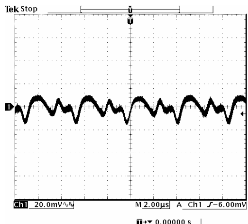
Vin=5 V, Vo=1.5 V
