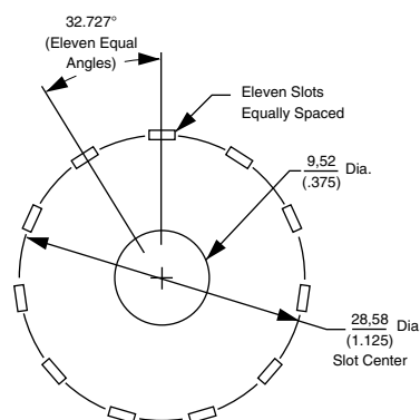
11R Socket
