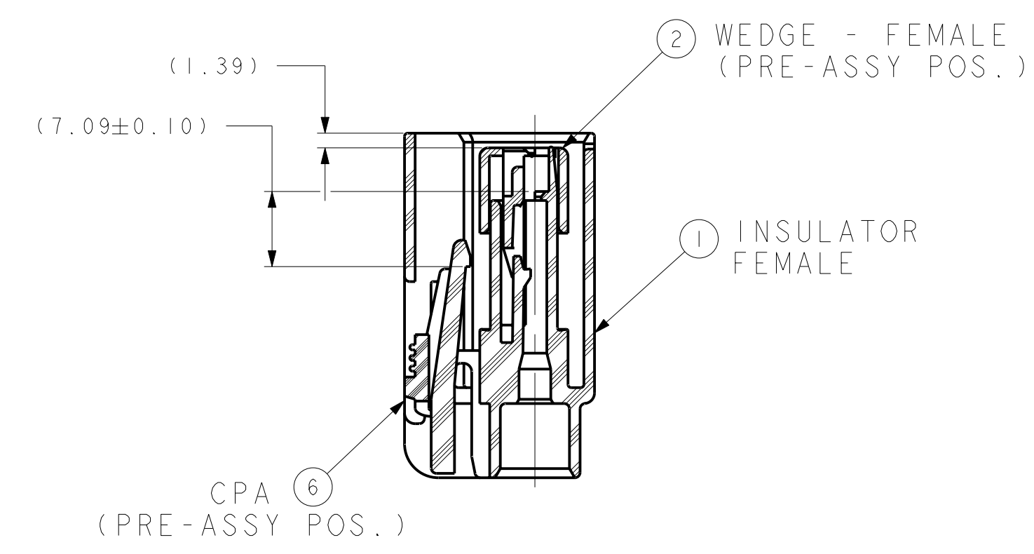
SECTION A-A
