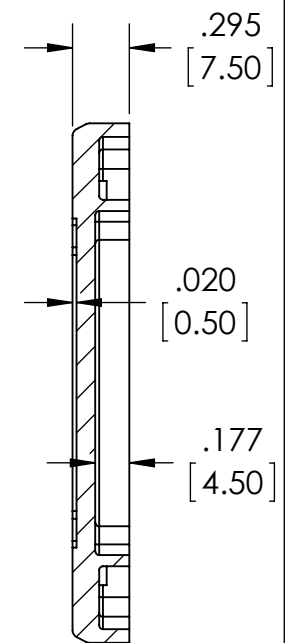
SECTION D-D
