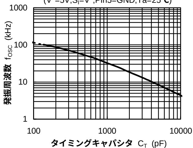
発振周波数対タイミングキャパシタ特性例
