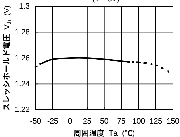
スレッシュホールド電圧温度特性例
