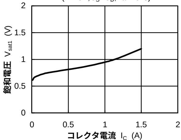
飽和電圧1対コレクタ電流特性例
