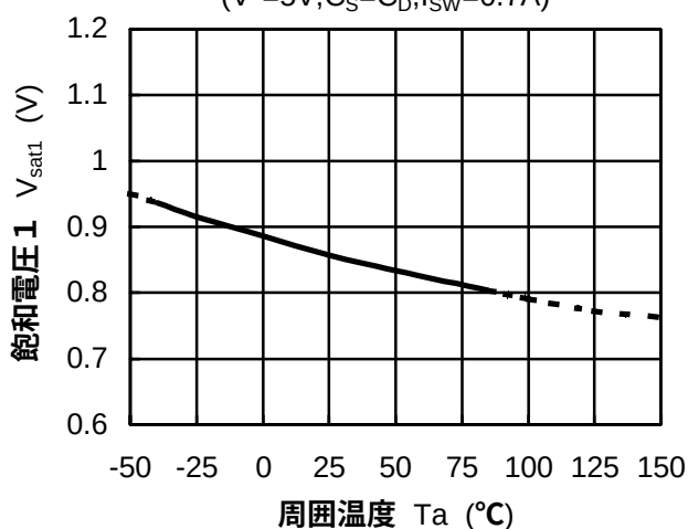
飽和電圧1 温度特性例
