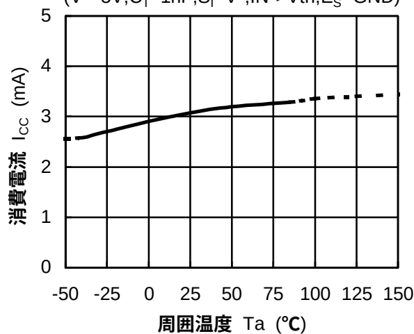
消費電流対温度特性例
