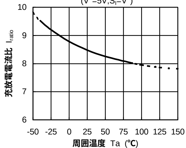
充放電電流比温度特性例
