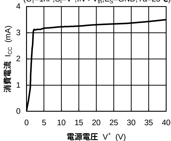
消費電流対電源電圧特性例
