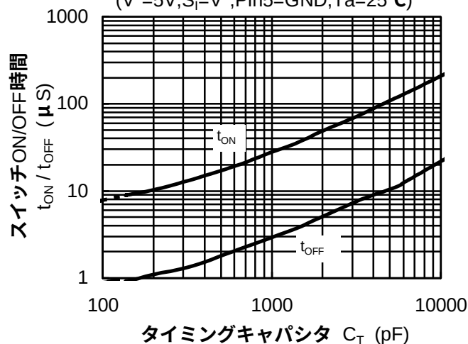
スイッチON/OFF時間対タイミングキャパシタ特性例
