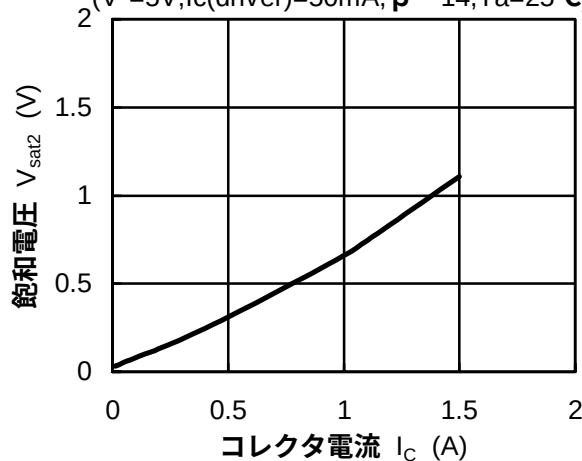
飽和電圧2対コレクタ電流特性例
