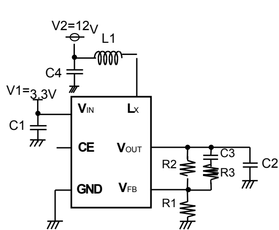
Fig 1. R1207N8xxA
