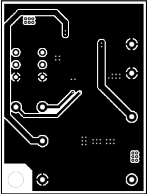
Fig.20 Bottom Layer
