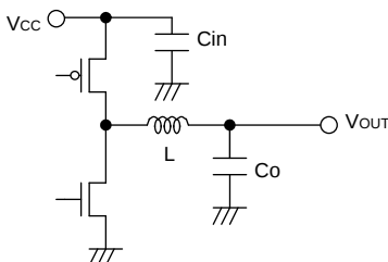
Fig.29 Input capacitor
