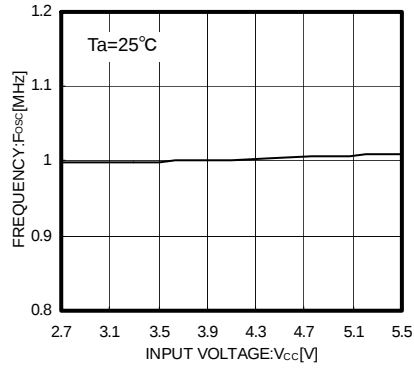
Fig.12 Vcc-Fosc
