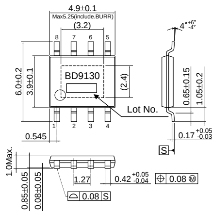
HTSOP-J8 (Unit:mm)
