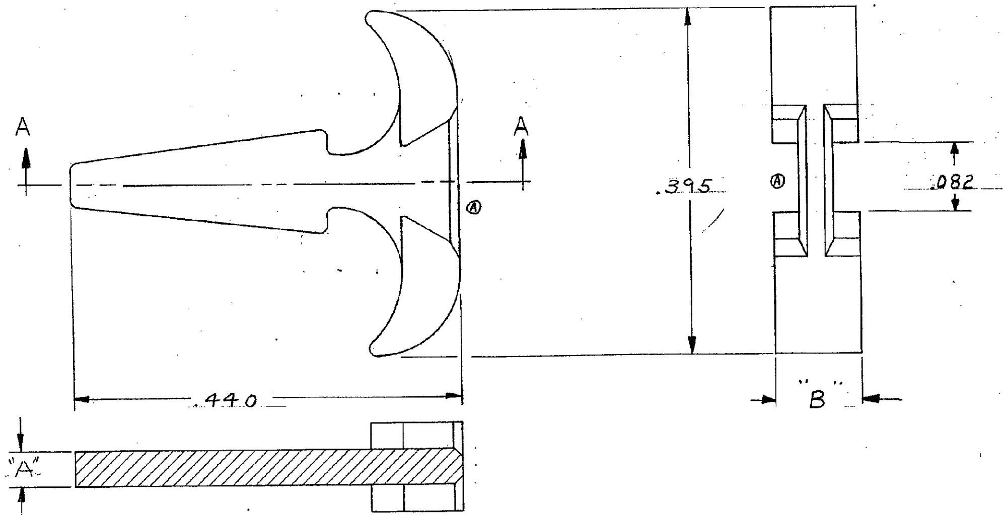
SECTION A-A
