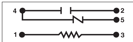
SPDT
