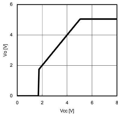
Fig.13 V_{cc} - V_o ( I_o=0\text{mA} )
