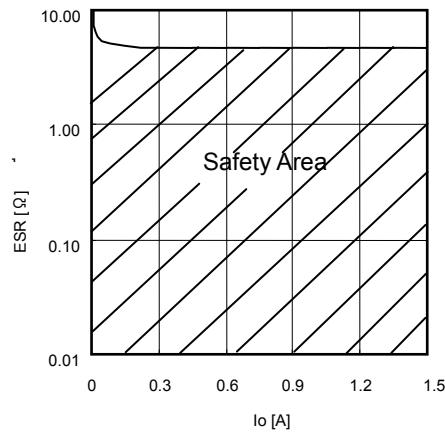
Fig.17 ESR condenser
