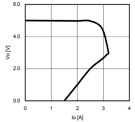
Fig.15 OCP
