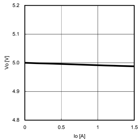
Fig.11 I_o - V_o
