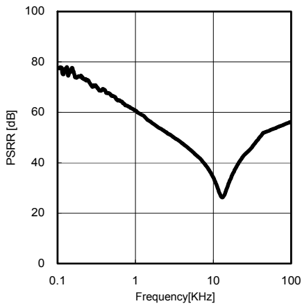
Fig.19 PSRR( I_o=0mA )
