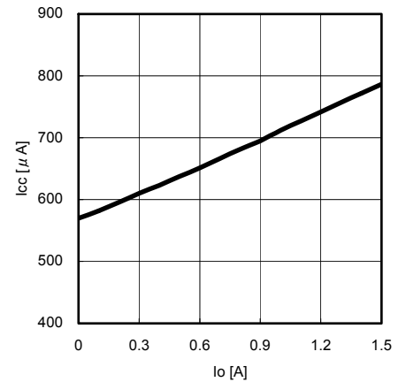
Fig.18 I_o - I_{cc}
