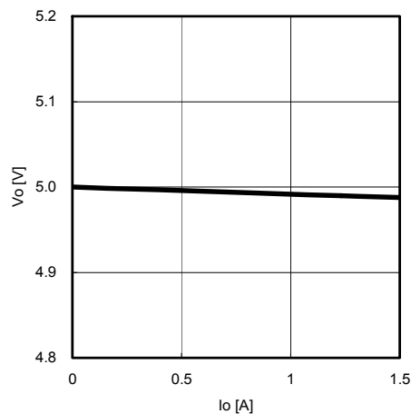
Fig.11 I_o - V_o
