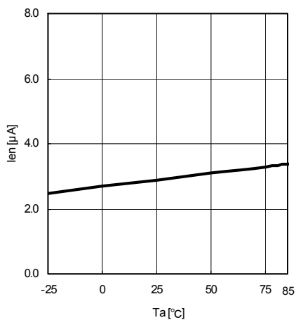
Fig.10 T_a - I_{EN}
