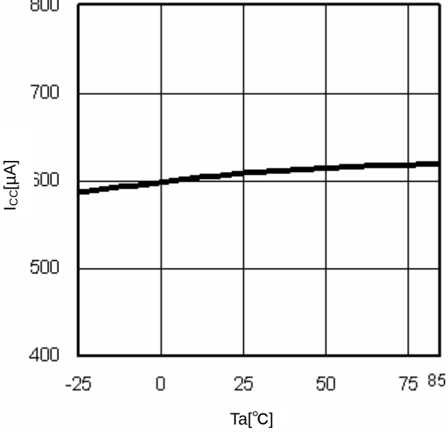
Fig.10 T_a-I_{cc}
