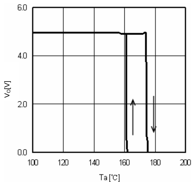
Fig.16 TSD ( I_O=0\text{mA} )
