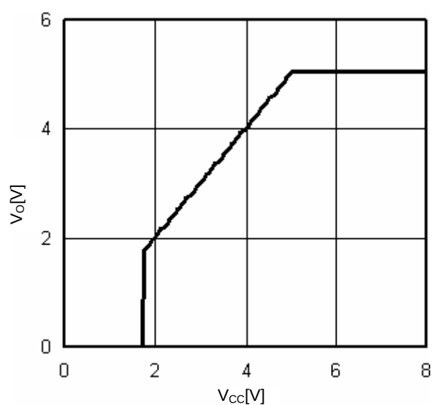
Fig.15 V_{CC}-V_O ( I_O=0\text{mA} )
