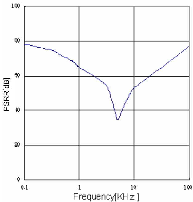
Fig.21 PSRR( I_o=0mA )
