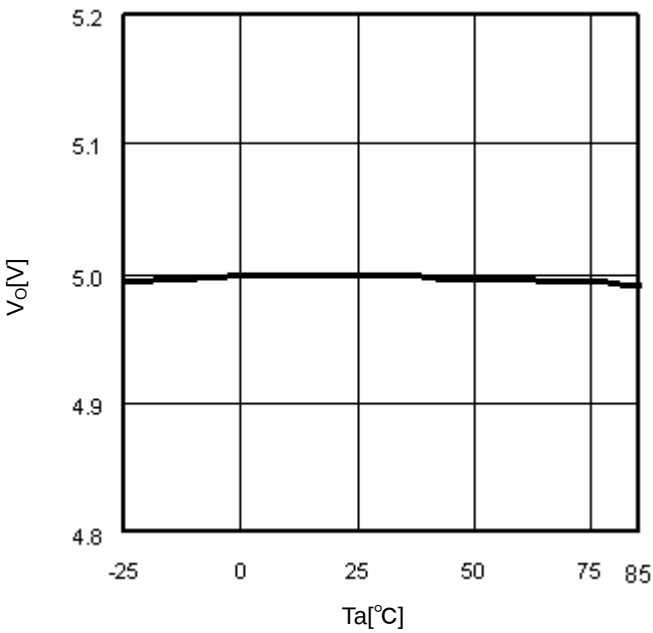
Fig.9 T_a-V_o ( I_o=0mA )
