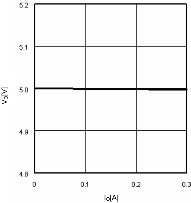
Fig.13 I O -V O
