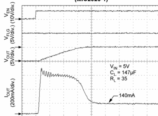
Turn-On (MIC2026-1)
