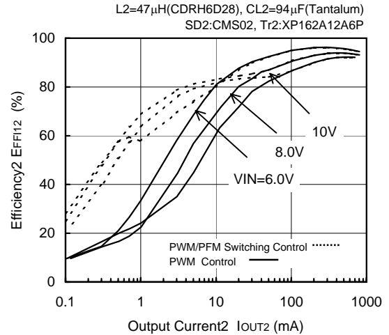
FOSC=180kHz, VOUT2=5.0V
