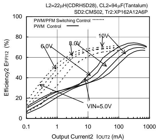
FOSC=300kHz, VOUT2=1.0V
