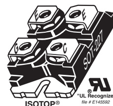
ISOTOP® APT46GA90JD40
