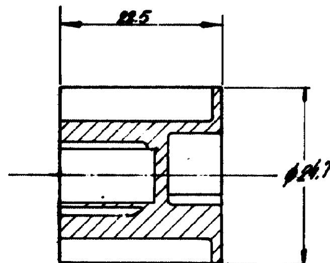
SECÇÃO AA
