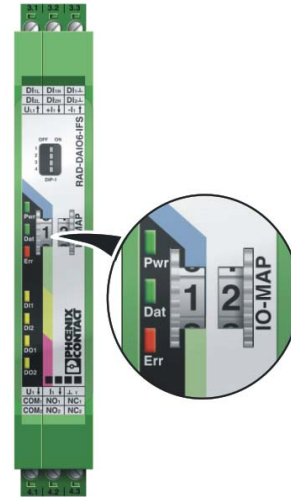
Bild 4 Thumb wheel
