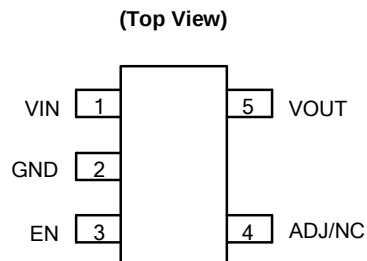
SOT25
