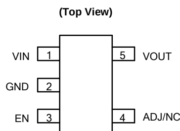
SOT25
