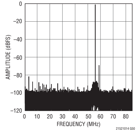
LTC2150-14: 32K Point FFT, f_{IN} = 571\text{MHz} , -1\text{dBFS} , 170\text{Mps}
