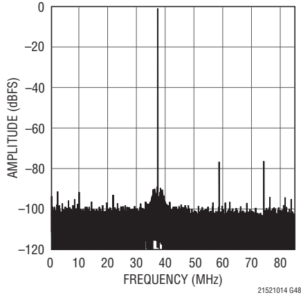
LTC2150-14: 32K Point FFT, f_{IN} = 380\text{MHz} , -1\text{dBFS} , 170\text{Mps}
