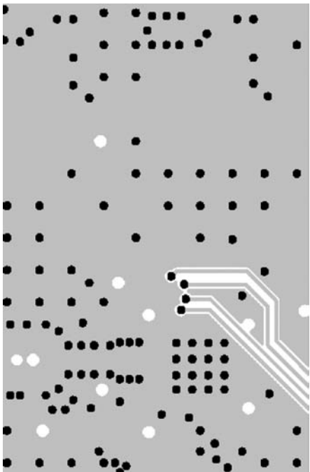
Inner Layer 3
