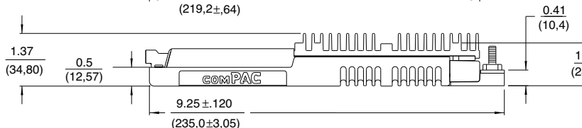
Optional heat sink (H1)
