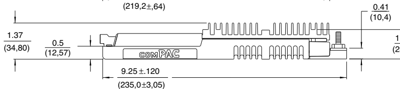
Optional heat sink (H1)
