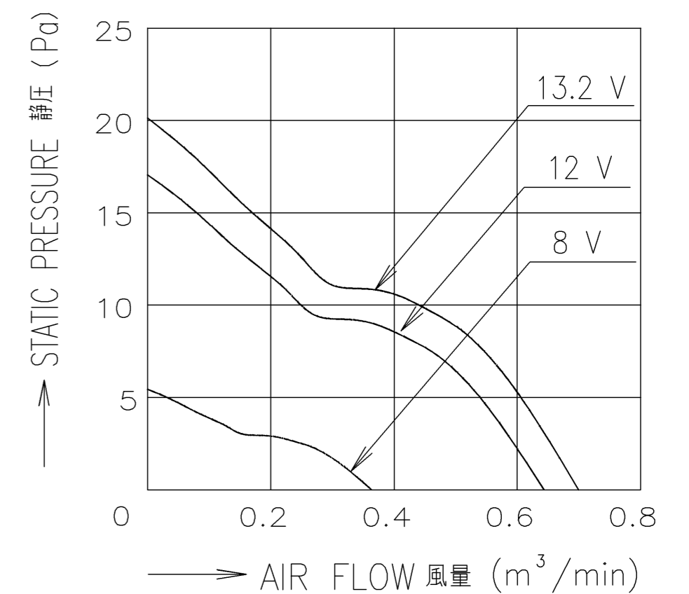
風量-静圧特性例
