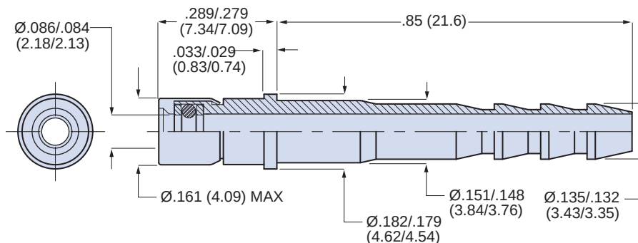
857-010 Socket Contact
