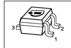
PG-SOT-323
