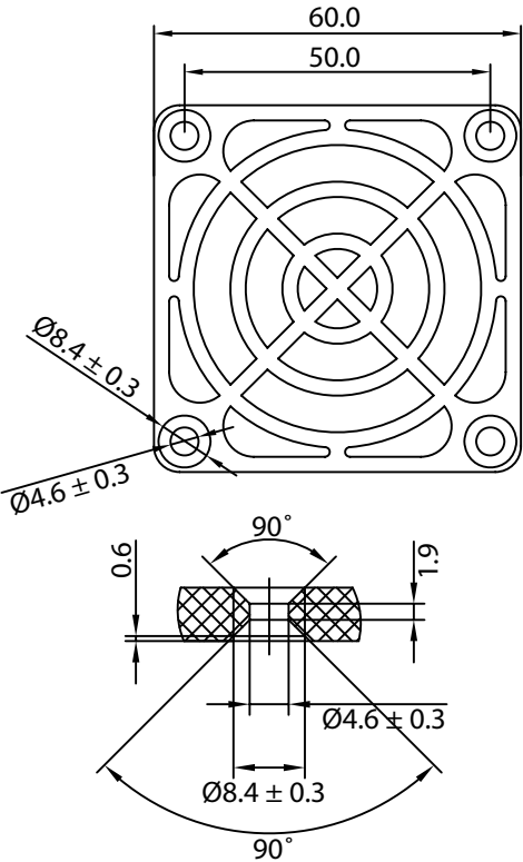
FAN GUARD
