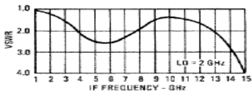
I-Port VSWR
