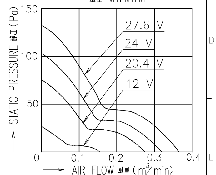
風量-靜圧特性例
