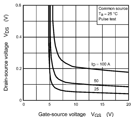
Fig. 8.4 V_{DS} - V_{GS}
