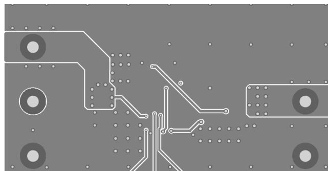
Inner Layer 2
