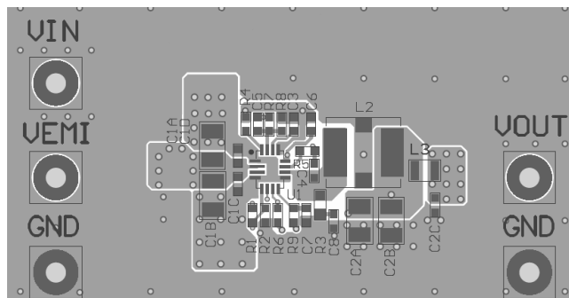
Top Layer
