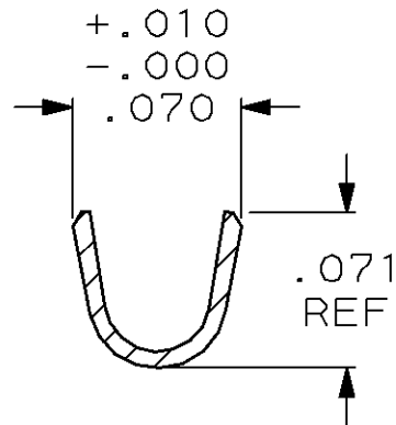
SECTION D-D
