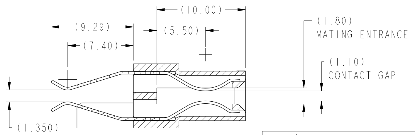
SECTION D-D
