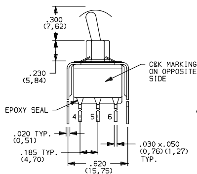
E201MD1__BE DPDT
