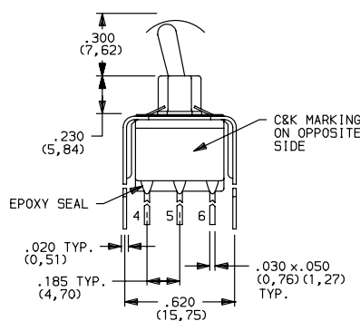
E201MD1__BE DPDT
