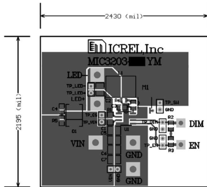
Top Layer
