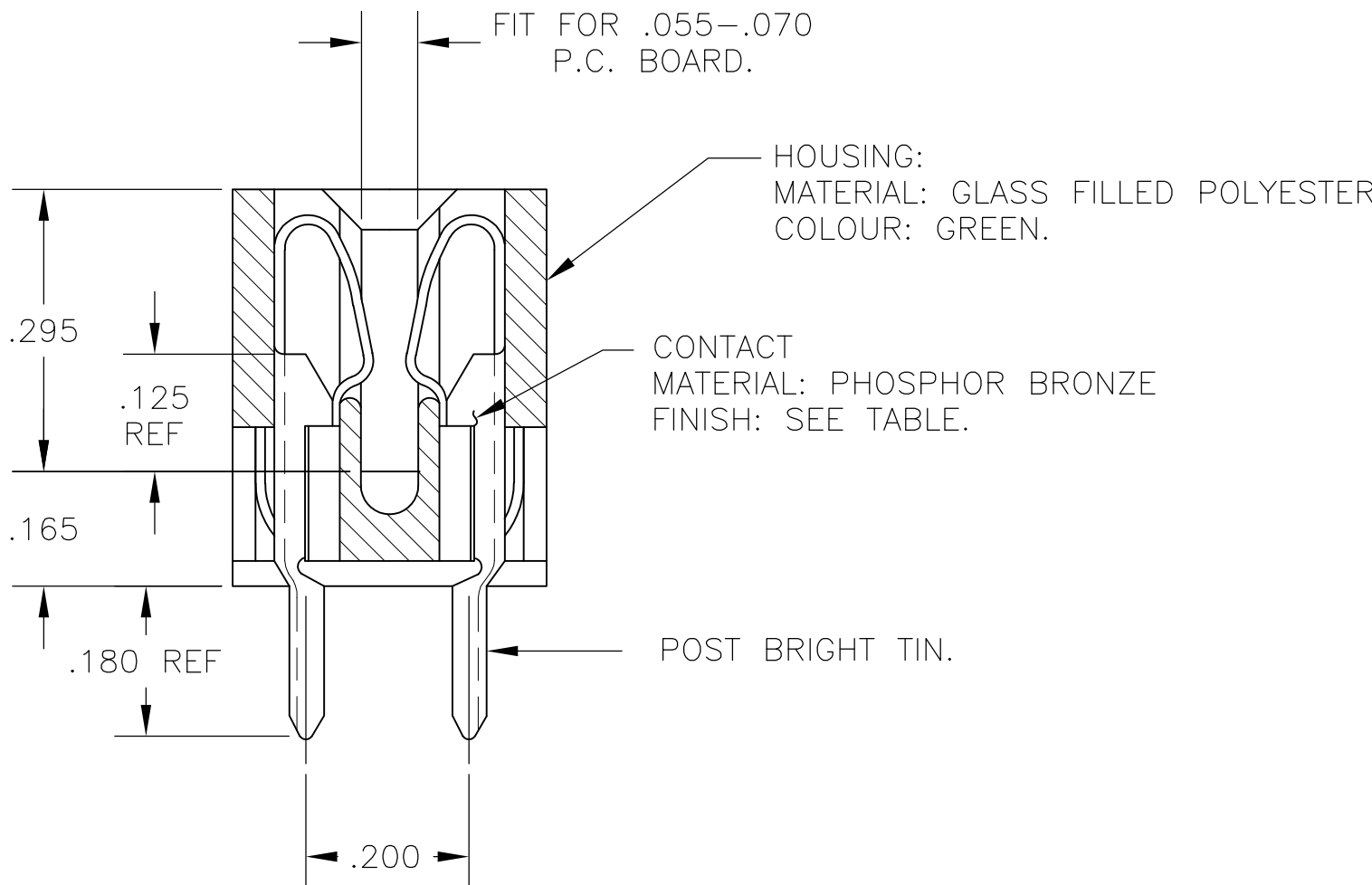
SECTION A-A
