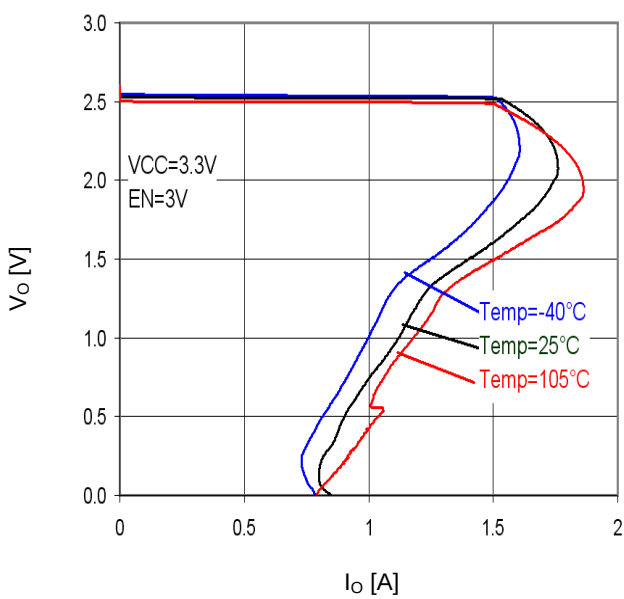
Figure 29. I_o - V_o
