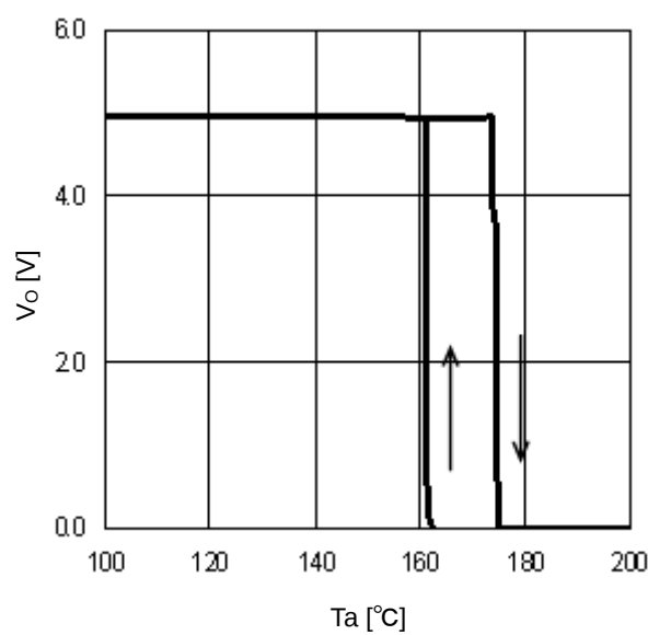
Figure 28. TSD ( I_o=0\text{mA} )
