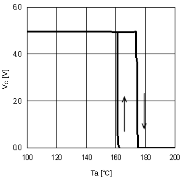
Figure 28. TSD ( I_o=0\text{mA} )
