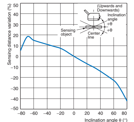
E3ZM-LS□4H(LS□9H)
