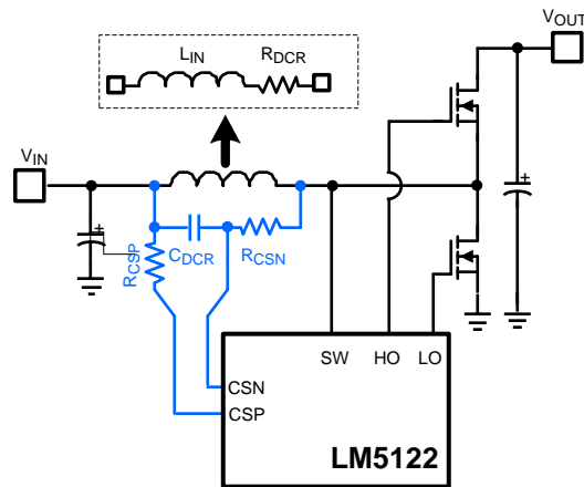
Figure 34. DCR Sensing
